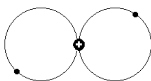
Wasserstoffatom im "2p"-Zustand
